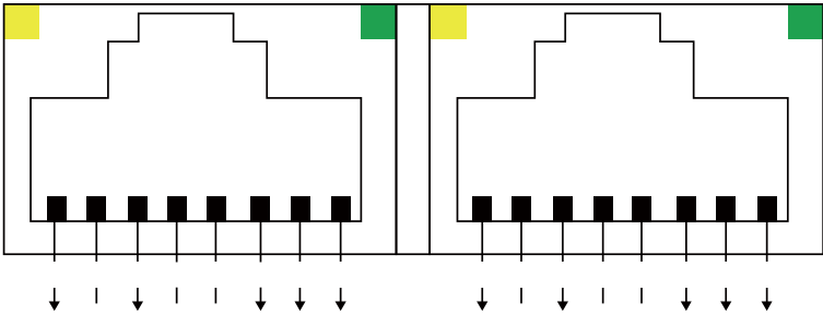
5-4 EtherCAT
