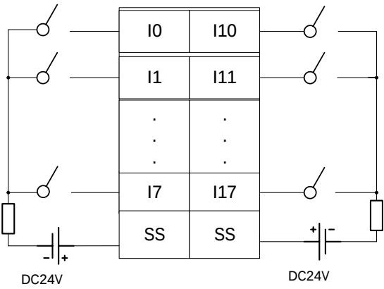
5-10 CN1
